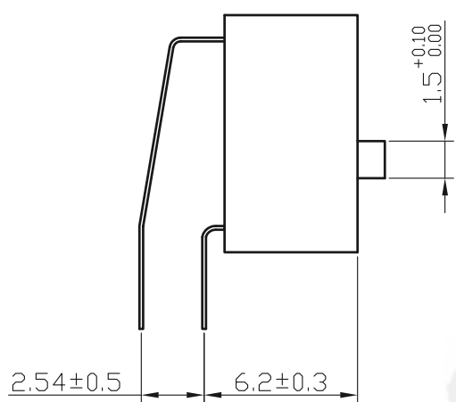
高推钮 (E)
