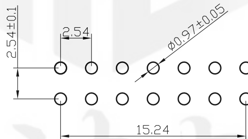
PCB开孔
