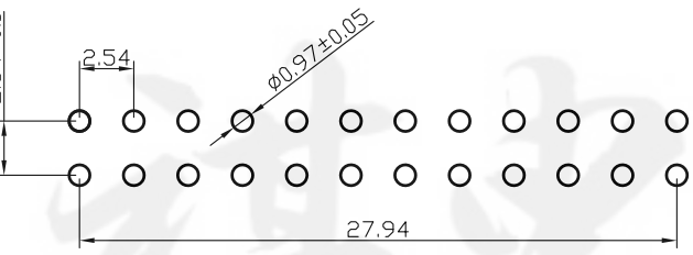
PCB开孔
