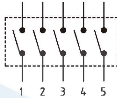
电路图
