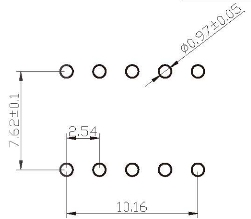
PCB开孔
