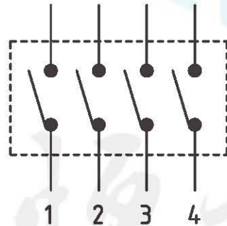
电路图
