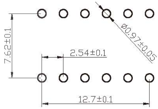
PCB开孔
