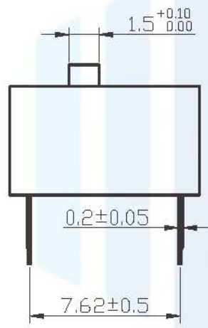
高推钮 (E)
