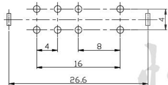
P.C.B LAYOUT
