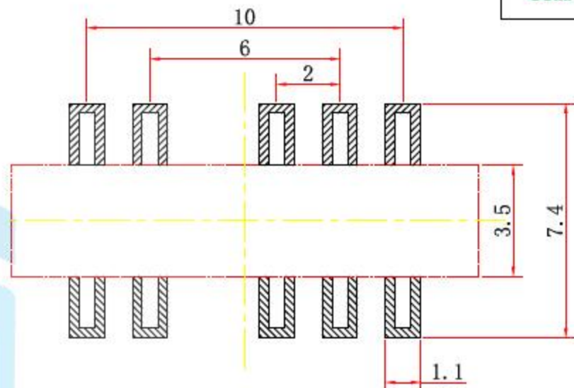
PCB板位置尺寸
