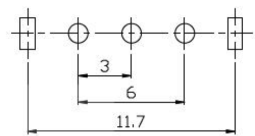
P.C.B LAYOUT
