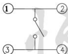
开关示意图
