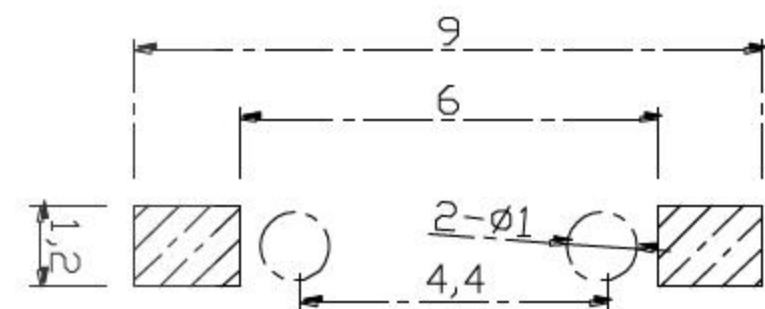
PCB. 焊接图
