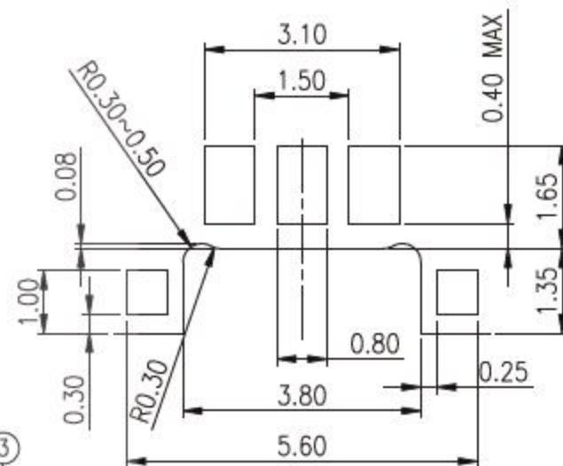
P.C.B. LAYOUT
