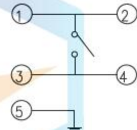
电路图
