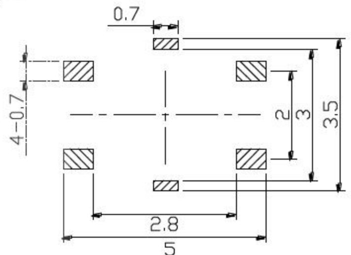
PCB. 焊接图
