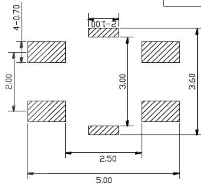
PCB. 焊接图
