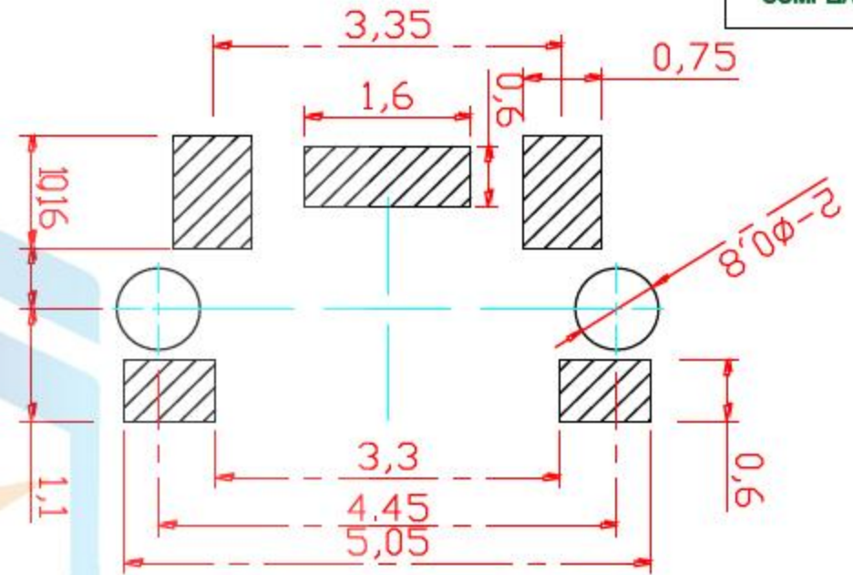
PCB. 焊接图
