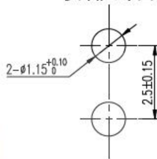
安装尺寸图
