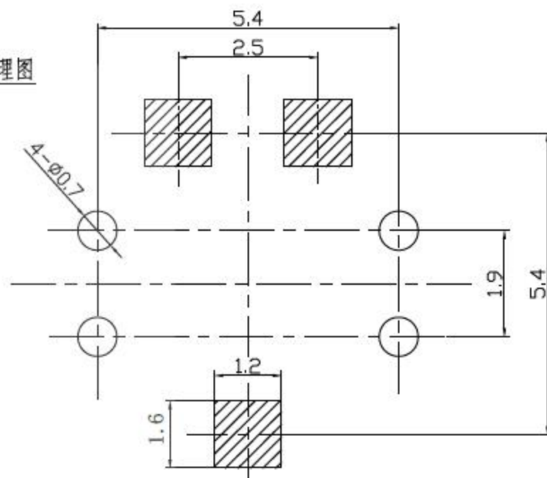
安装尺寸图
