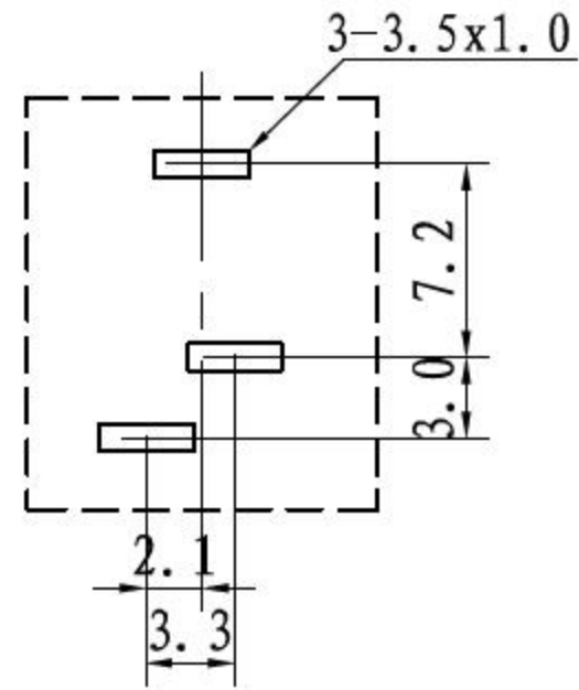
线路板安装尺寸示意图
