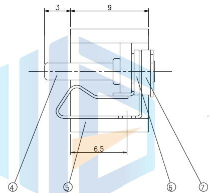
接点示意图
