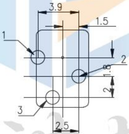
线路板开孔
