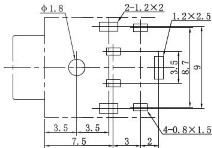
印刷电路板开孔尺寸
