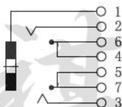
按点示意图
