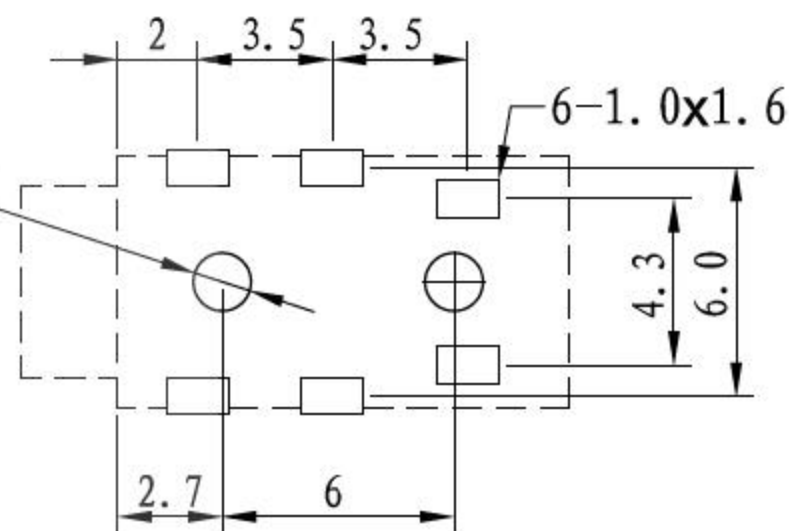
尺寸安装线路板示意图
