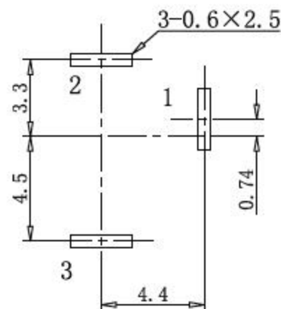
印制线路板开孔尺寸
